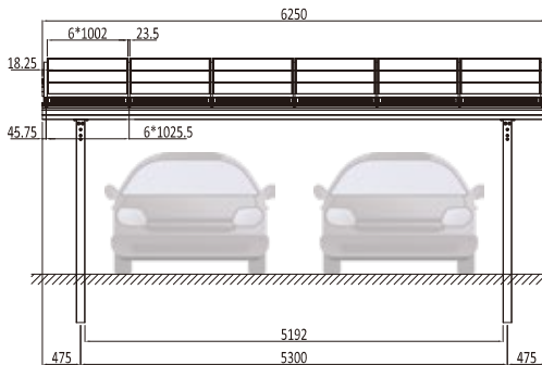
SPT-G2P-330H 正面外形図
