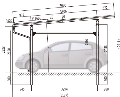
SPT-G2/4/6/8P-330H 側面外形図
