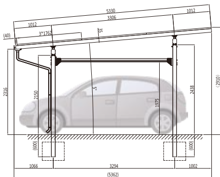
SPT-G2/4/6/8P-470H 側面 外形図
