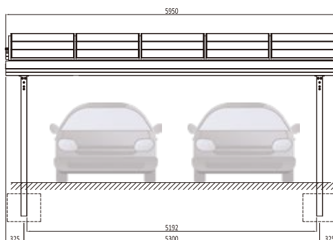
SPT-G2P-470H 正面 外形図
