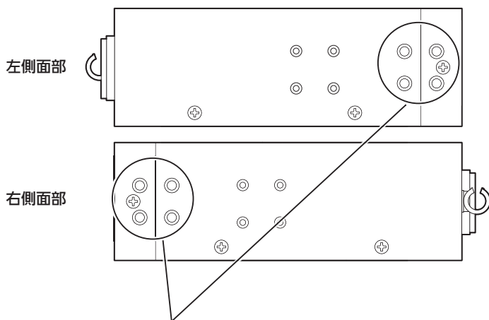
19 インチラックマウント用 金具取り付けねじ穴
