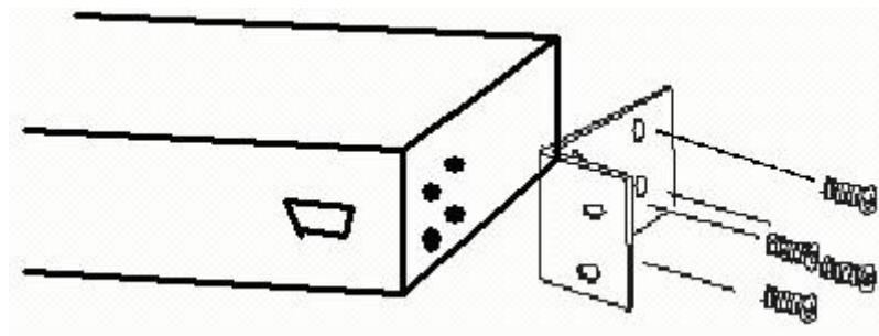
図2-1 19インチラックへの設置
