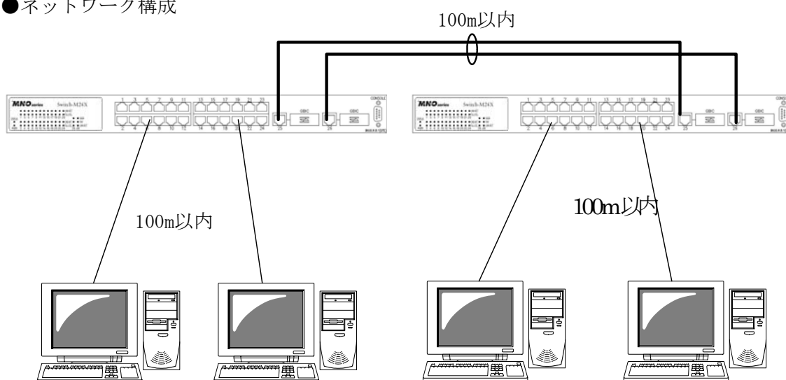
図3-1 接続構成例
