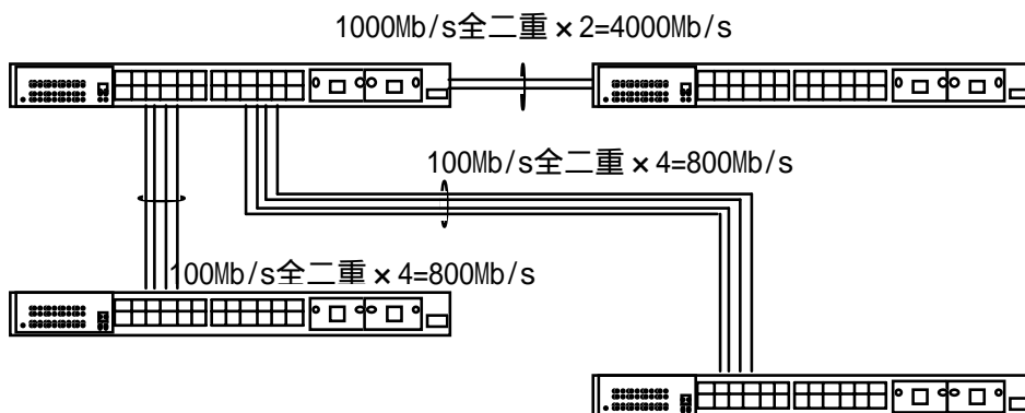
図4-24 トランキングを用いた構成例2
