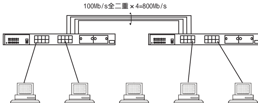
図4-23 トランキングを用いた構成例 1
