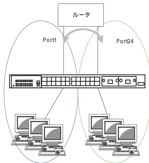
図5-1 ブロードキャストドメインの分割
