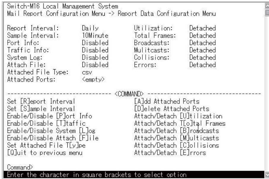
図4-16 メールの内容の設定 (Report Data Configuration Menu)
