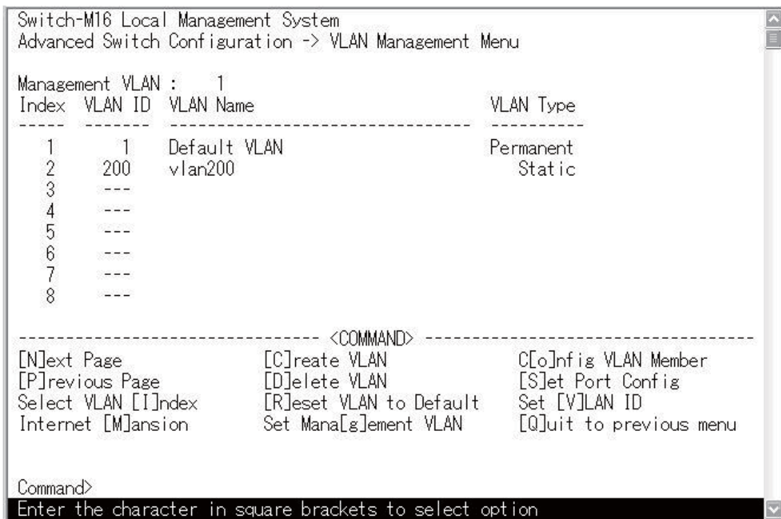
図4-20 VLAN設定メニュー (VLAN Management Menu)
