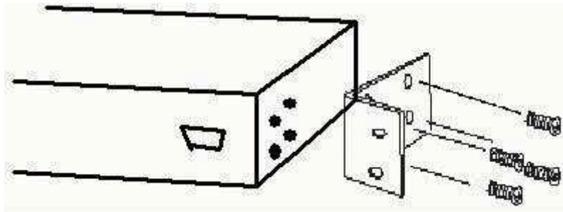
図2-1 19インチラック設置時の金具取付
