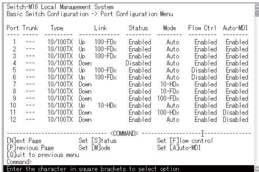
図4-11 各ポートの設定(Port Configuration)
