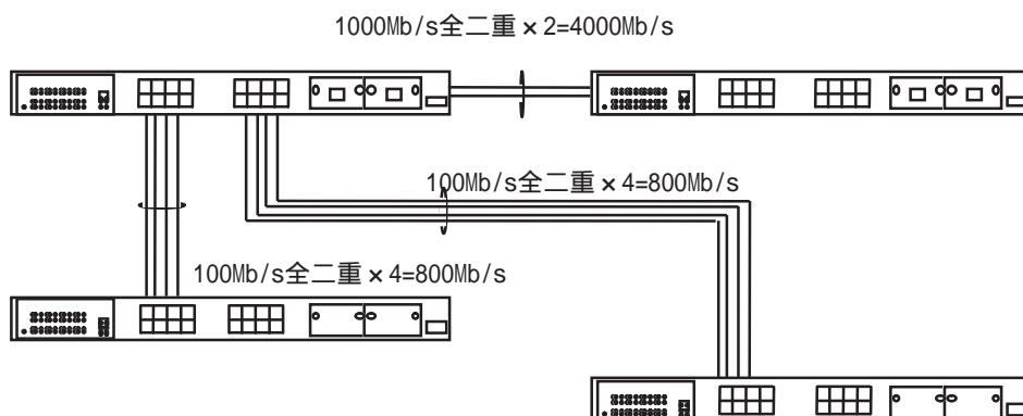
図4-24 トランキングを用いた構成例 2
