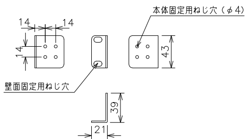
壁取付用金具 (別売: PN71053)
