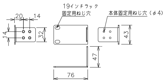
取付金具 (19インチラックマウント用) (同梱)
