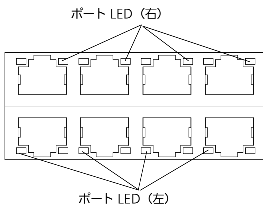
図 1-2 ポート LED
