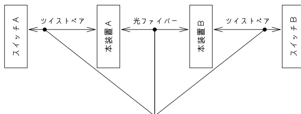
各々のリンクが確立した場合にリンクLEDが点灯します
