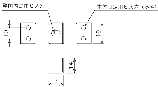
壁面取付金具 (添付)
