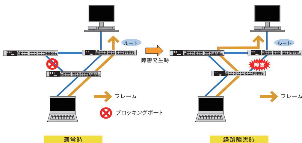
図 72-1 リングプロトコルの概要
