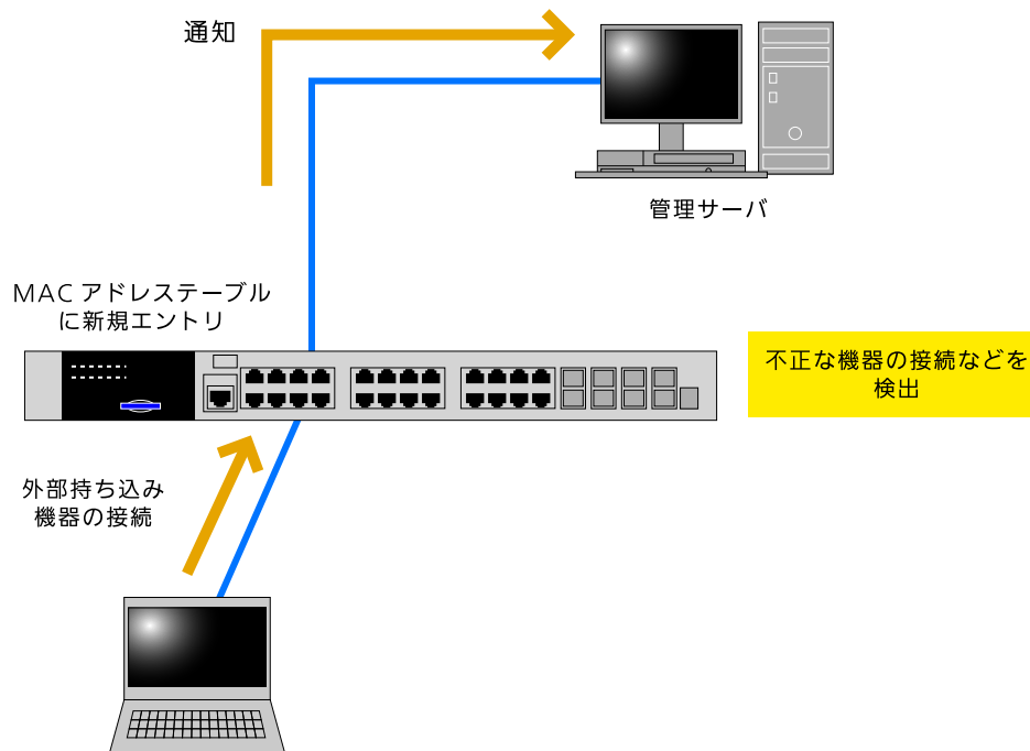
図 50-1 MAC Notification の概略
