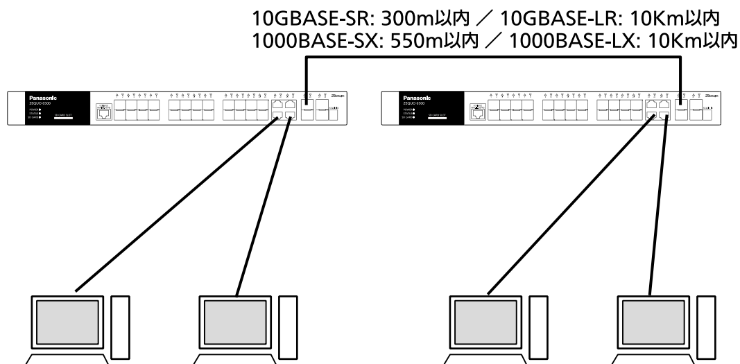
図 3-3 光ファイバケーブル接続例
