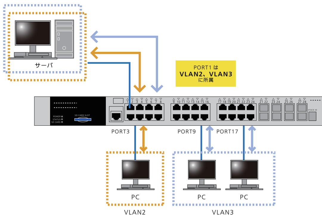
図 11-1 Asymmetric VLAN の概略
