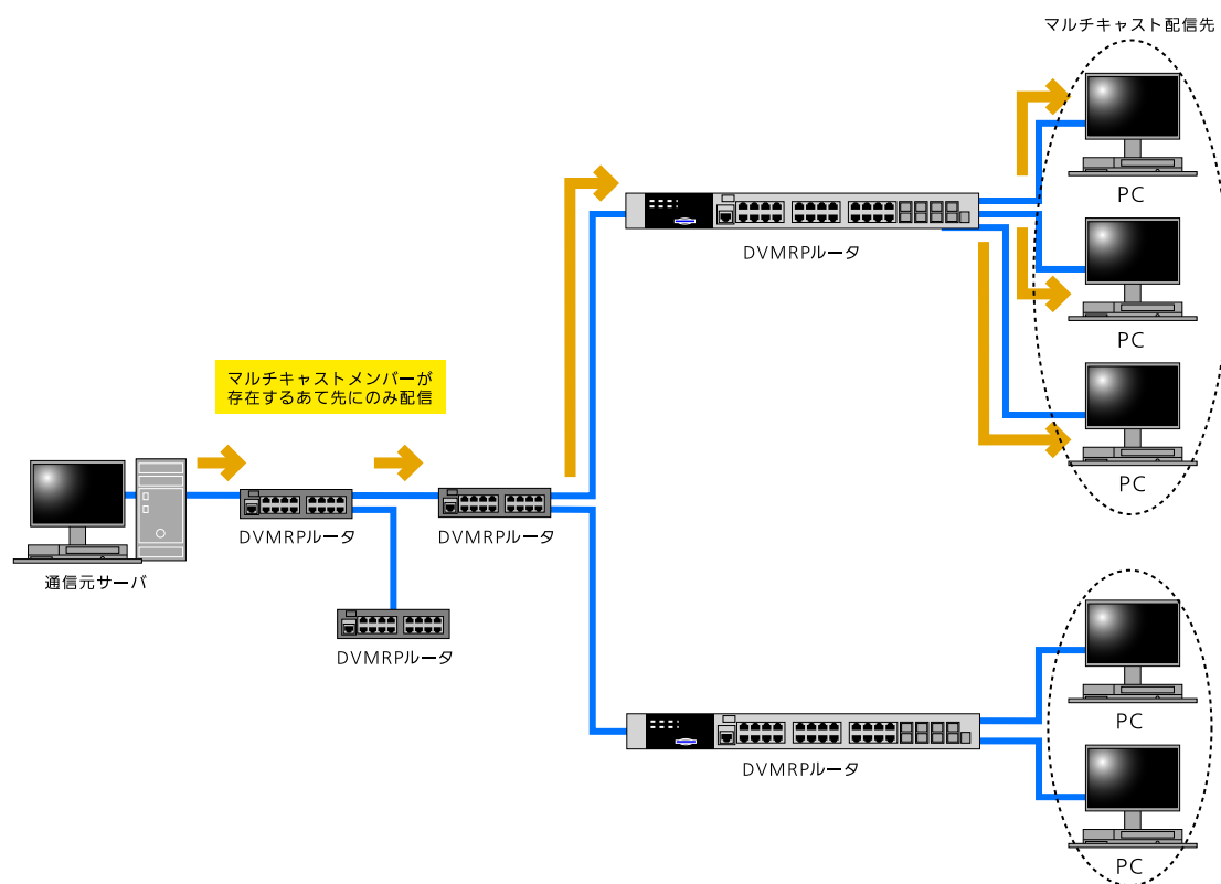
図 28-1 DVMRP によるルーティング
