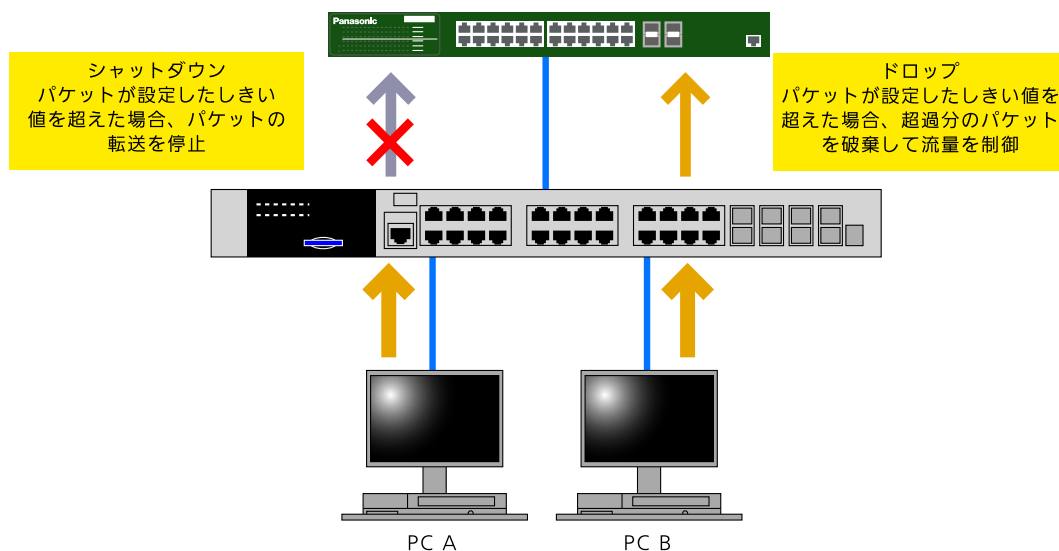
図 63-1 パケットストームの制御
