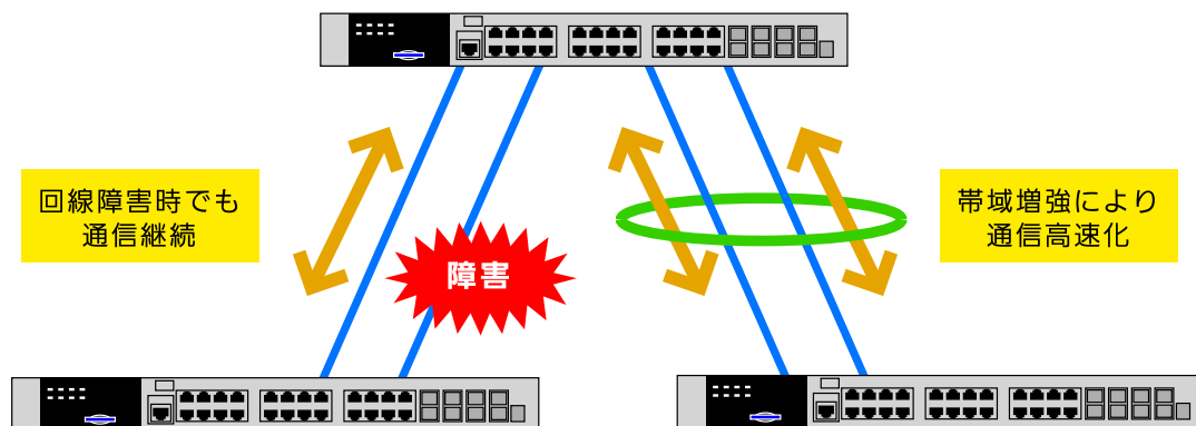
図 47-1 リンクアグリゲーションの概略
