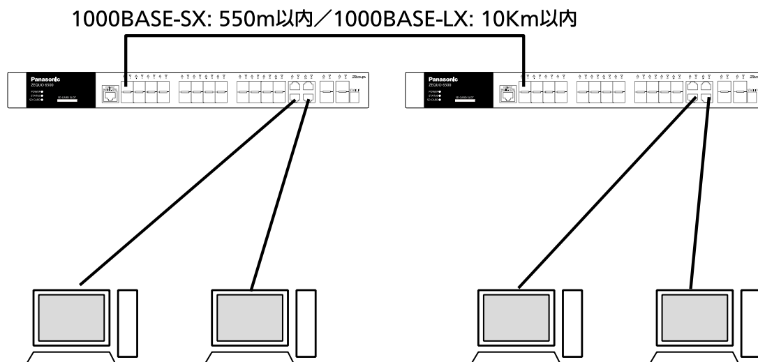
図 3-1 光ファイバケーブル接続例
