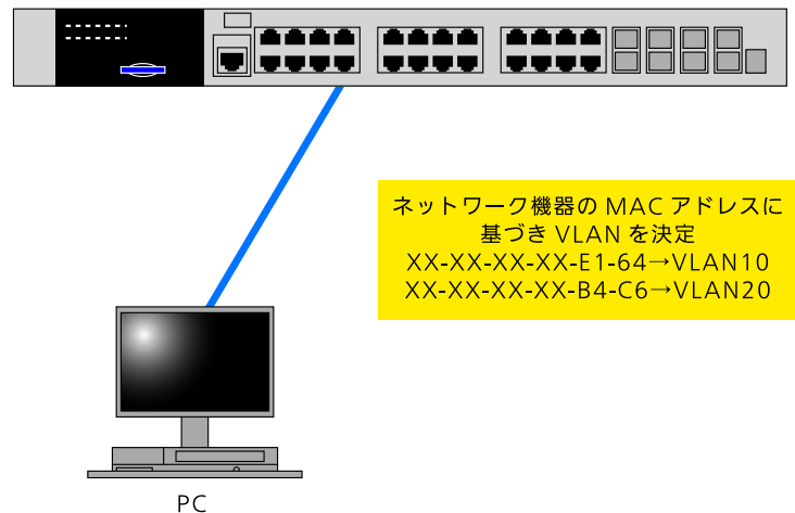
図 79-1 Static MAC-based Subnet VLAN の概略
