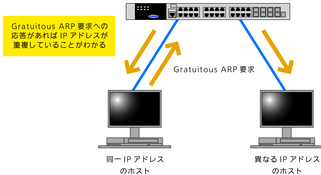
図 34-1 Gratuitous ARP の概略
