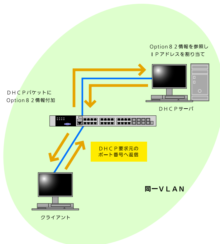
図 22-1 DHCP Local Relay の概略
