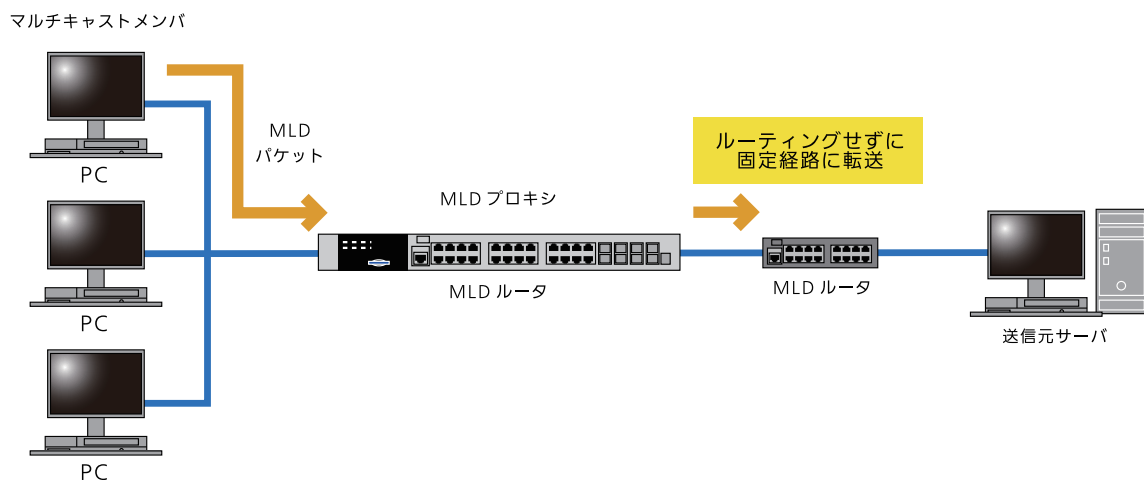
図 54-1 MLD プロキシの概略
