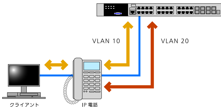
図 88-1 Voice VLAN の概略
