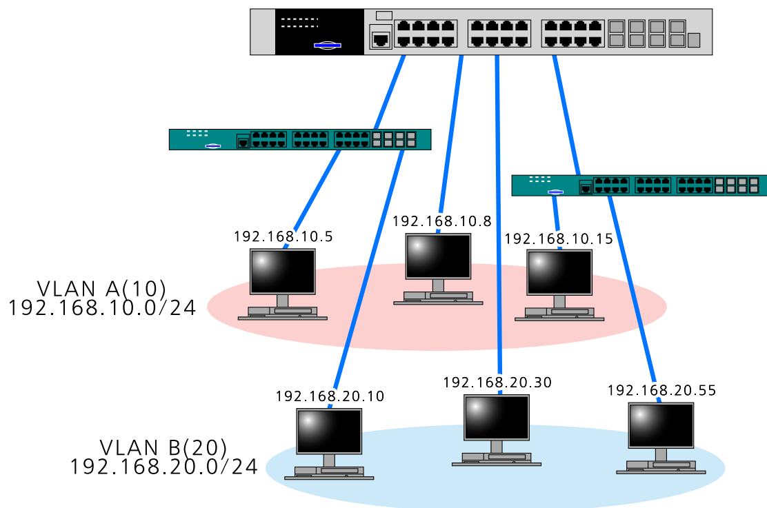
図 80-1 Subnet VLAN の概略
