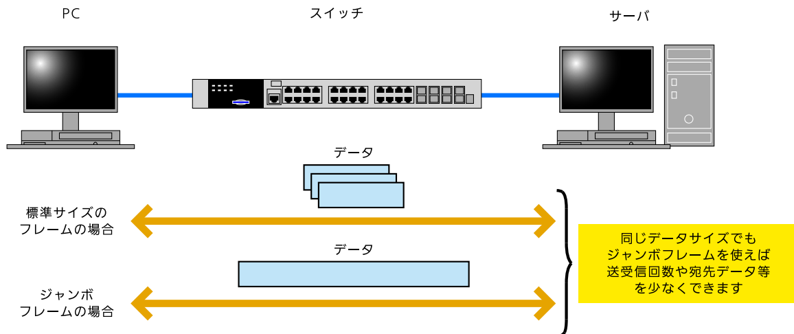
図 43-1 ジャンボフレーム概略
