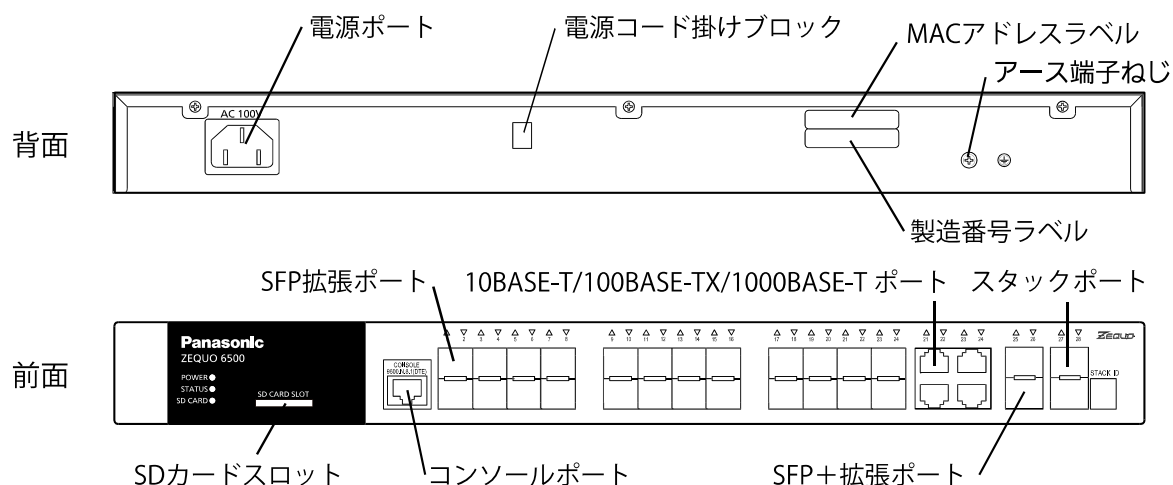
図 1-1 背面、前面
