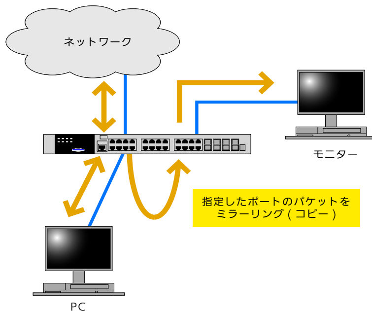
図 53-1 ミラーリングの概要
