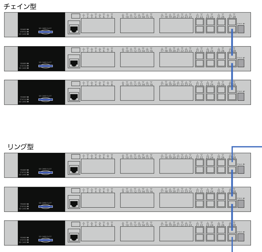
図 78-1 チェーン型、リング型のスタッキング
