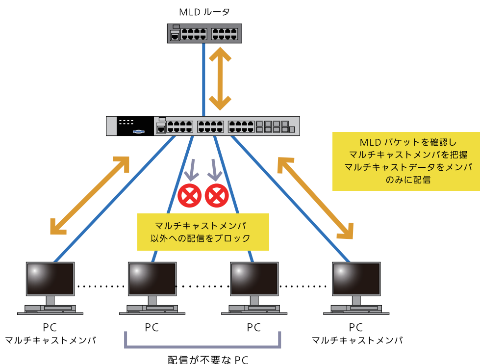
図 55-1 MLD Snooping の概略
