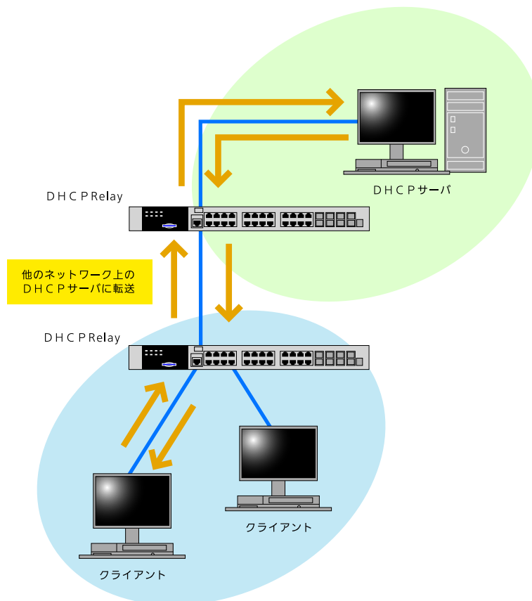
図 23-1 DHCP Relay の概略
