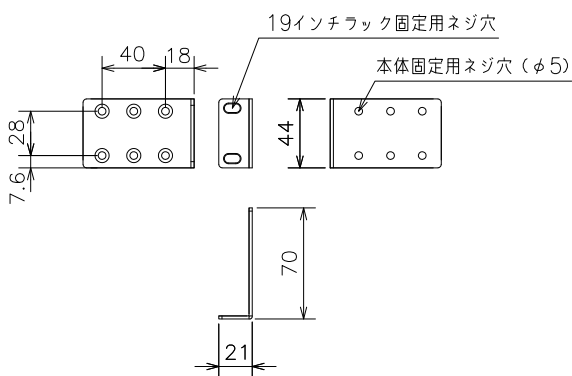
19インチラック固定用具 (同梱)
