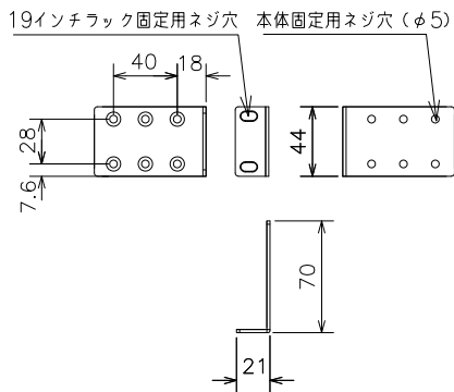
19インチラック固定用金具 (同梱)
