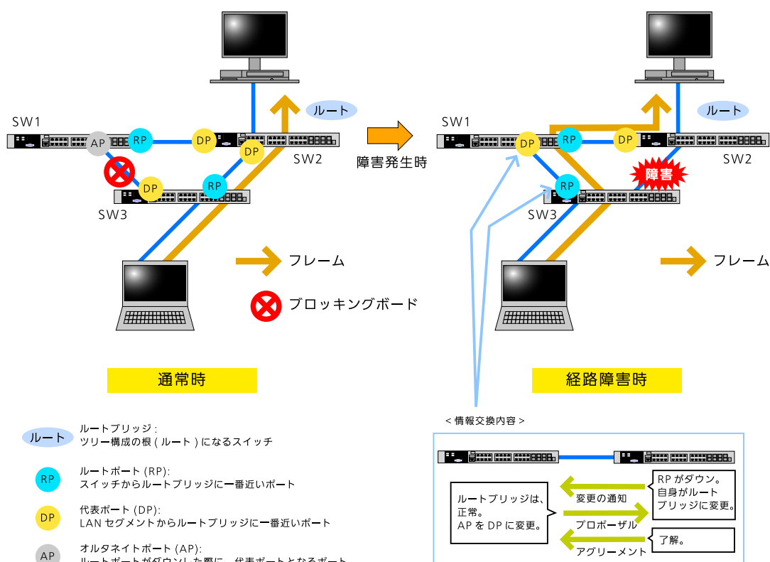
図 57-2 RSTP の概略
