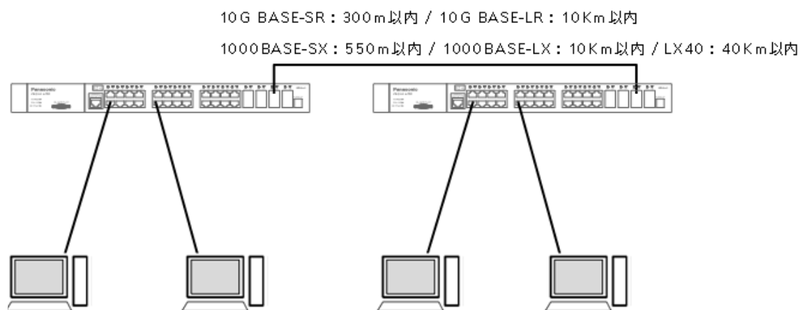
図 3-3 光ファイバケーブル接続例
