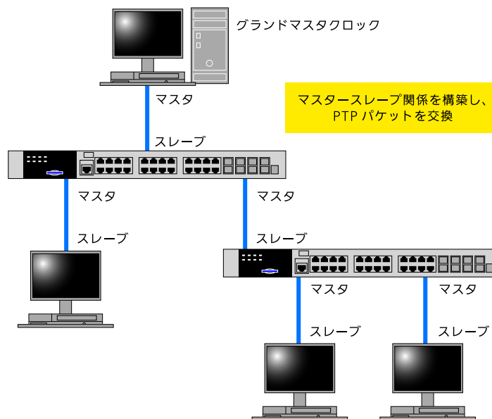
図 52-1 PTP の概略
