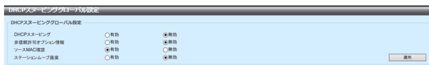
図 9-41 DHCP スヌーピンググローバル設定
