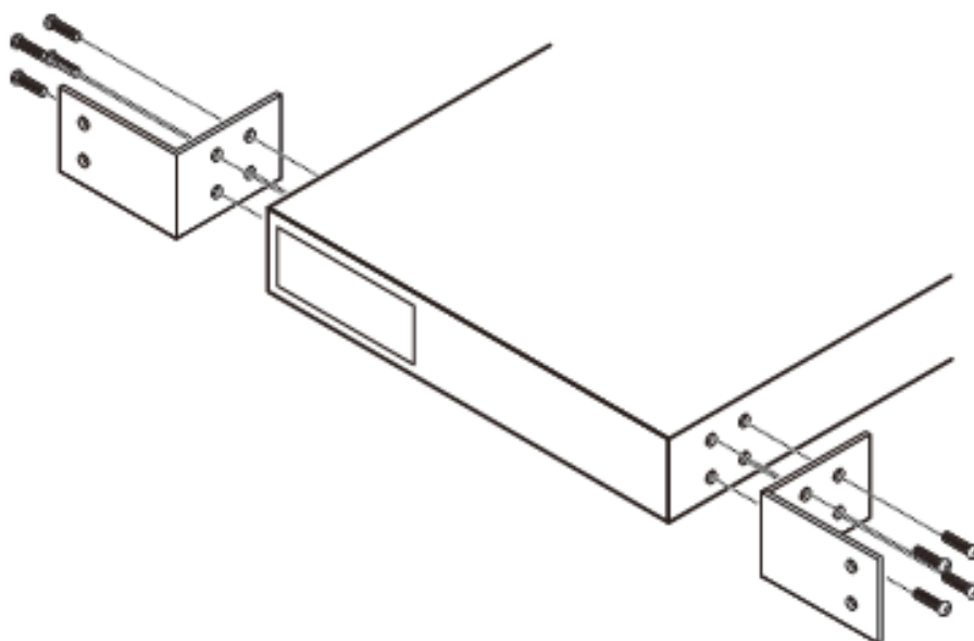
図 2-2 ラックへの設置
