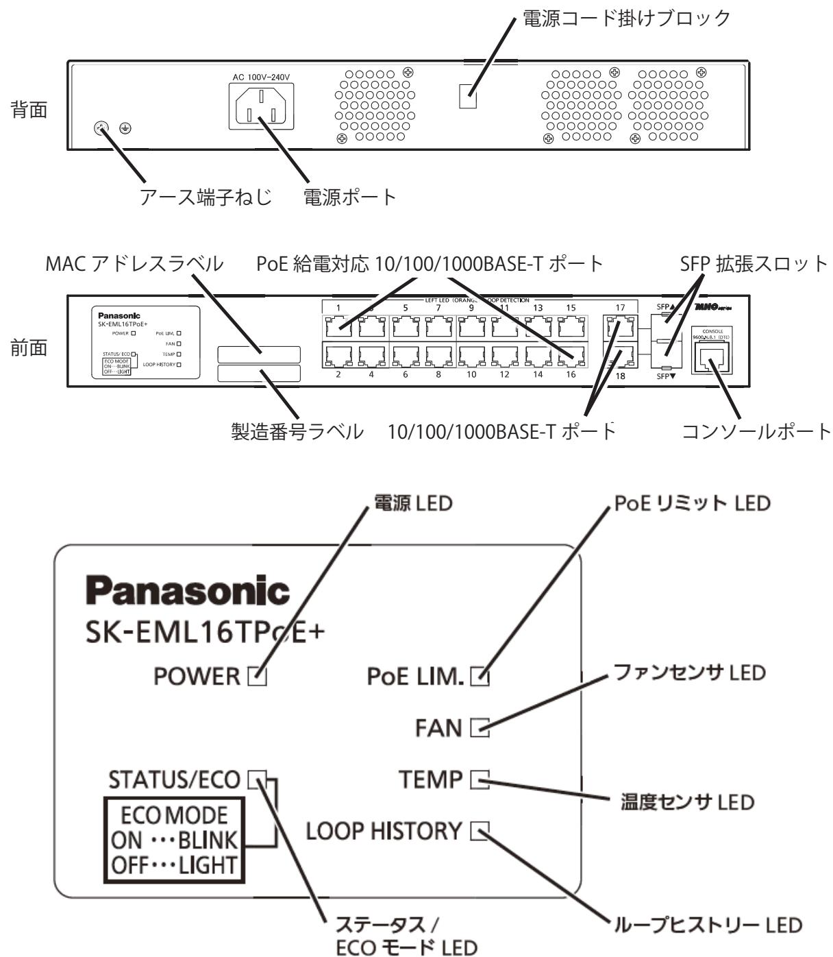
図 1-1 各部の名称
