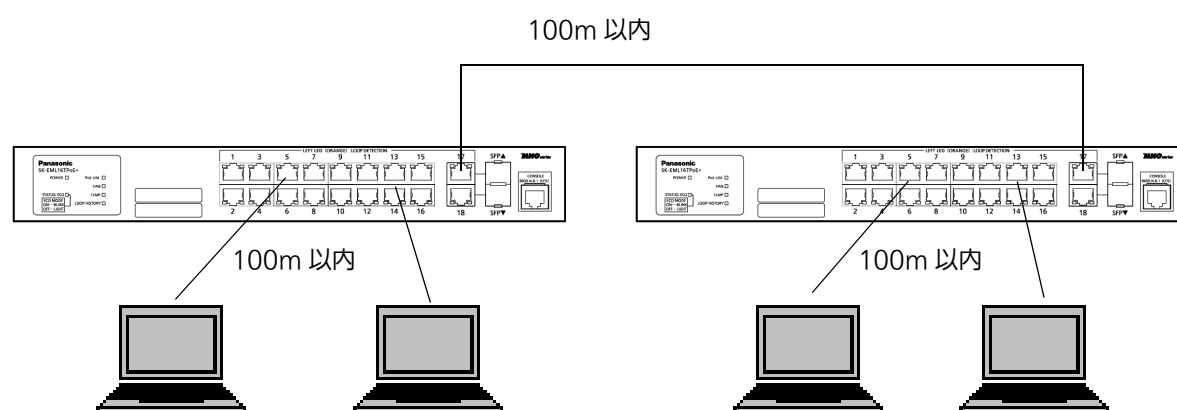
図 3-1 接続構成例
