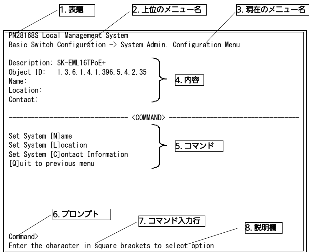
図 4-2 画面構成
