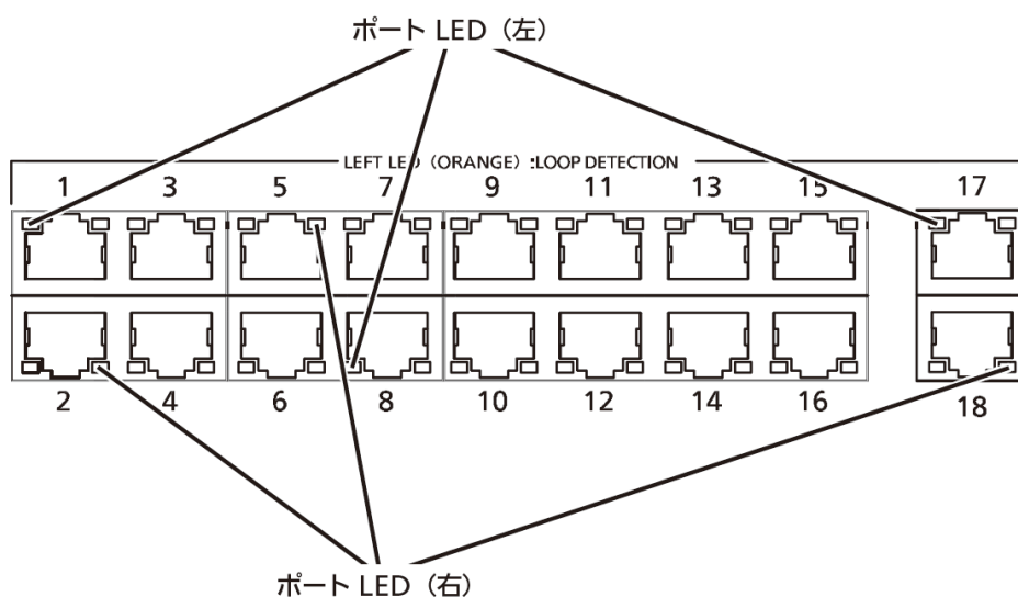
図 1-2 ポート LED
