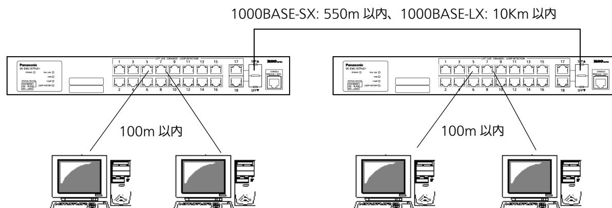
図 3-2 光ファイバケーブル接続例
