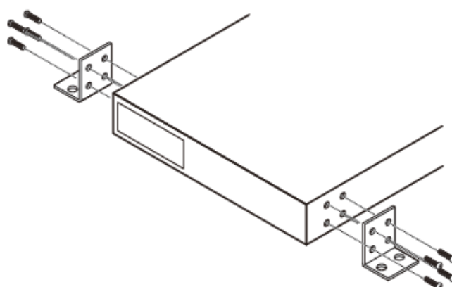
図 2-3 壁面への設置
