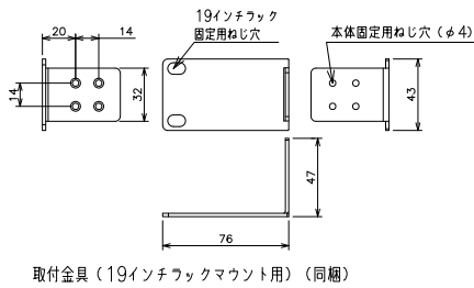
取付金具（19インチラックマウント用）（同梱）
