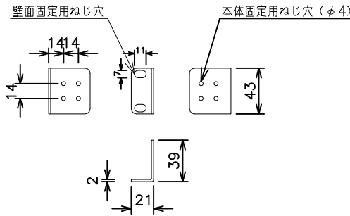
取付金具（壁取付用）（同梱）
