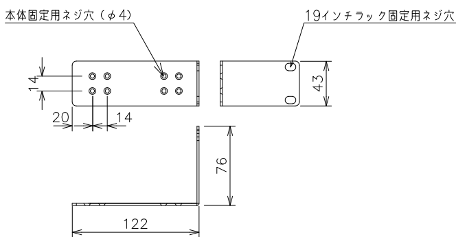
取付金具 (19インチラックマウント用) (同梱)
