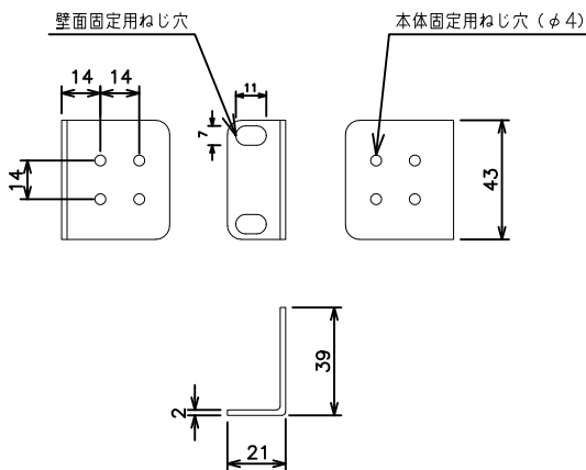
取付金具 (壁取付用) (同梱)
