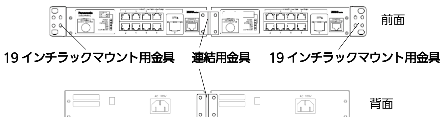
図 2-2 19 インチラックへの設置
