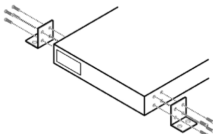
図 2-3 壁面への設置
