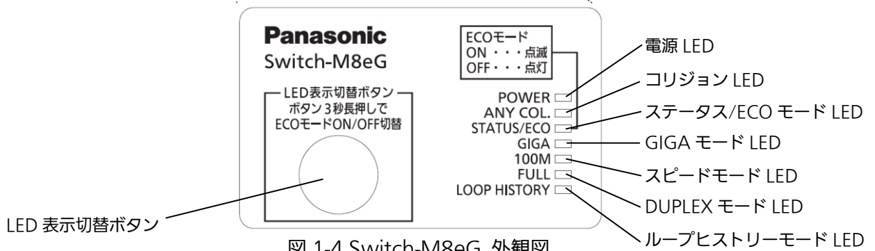
図 1-4 Switch-M8eG 外観図
