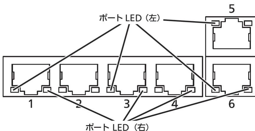
図 1-5 ポート LED
