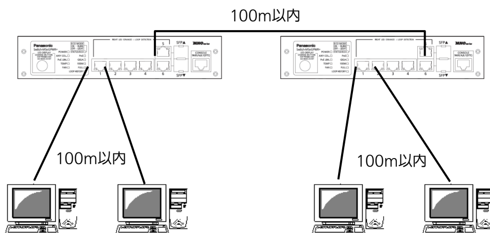
図3-1 接続構成例
