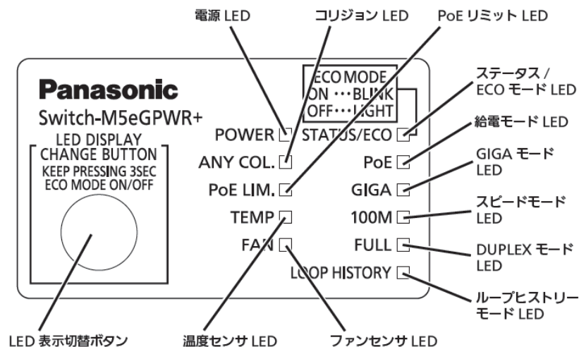
図 1-2 前面LED拡大図
