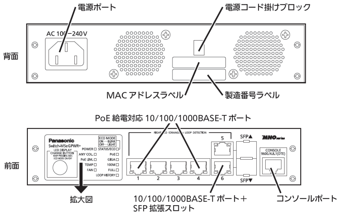
図 1-1 Switch-M5eGPWR+
