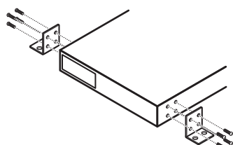
壁取付用金具の接続
