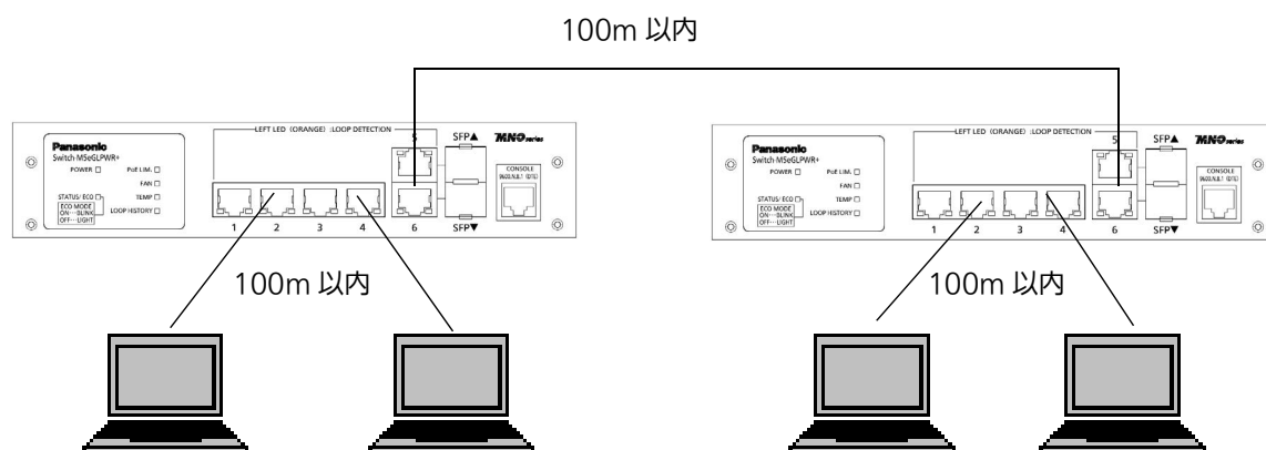
図 3-1 接続構成例
