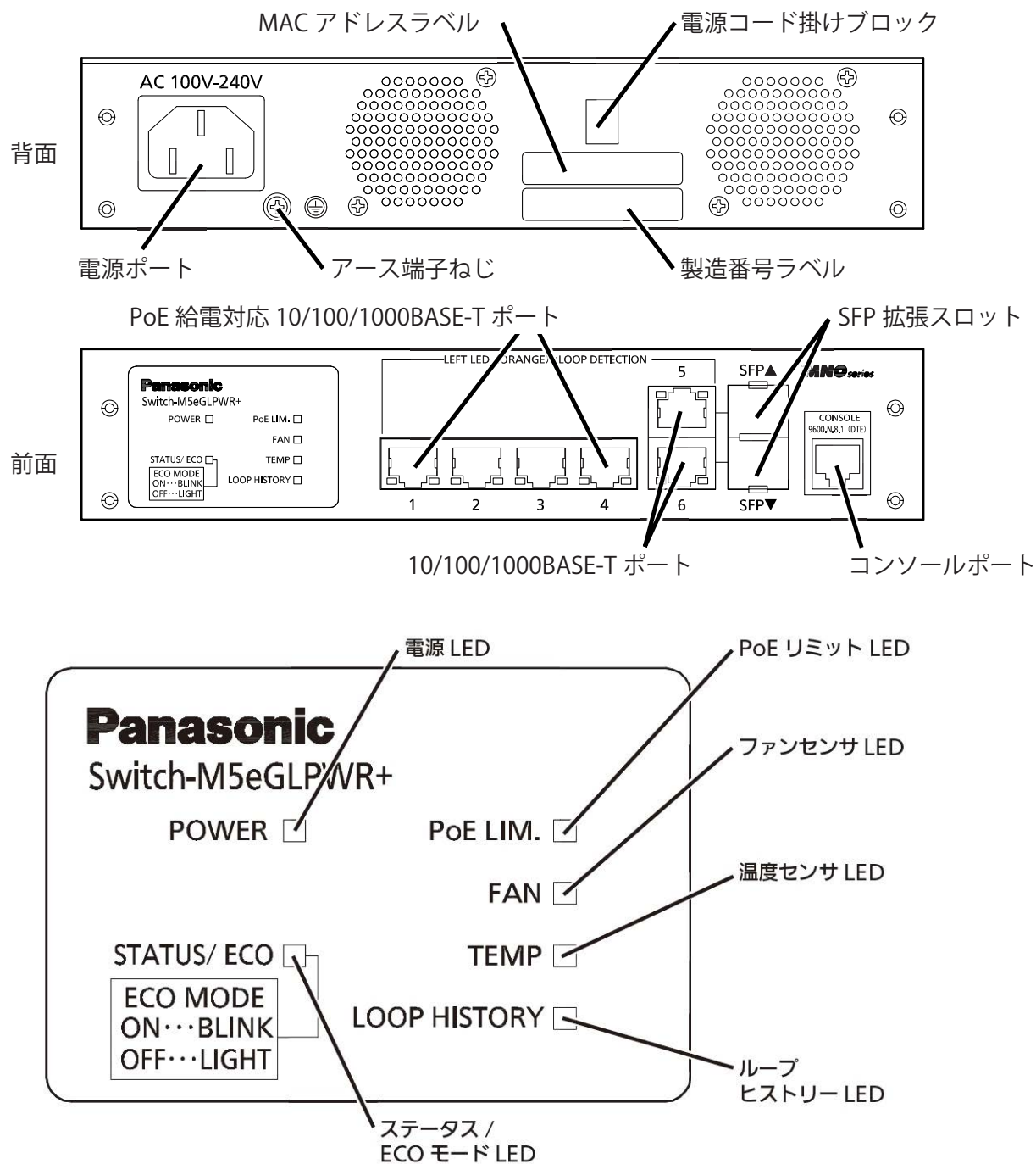
図 1-1 各部の名称
