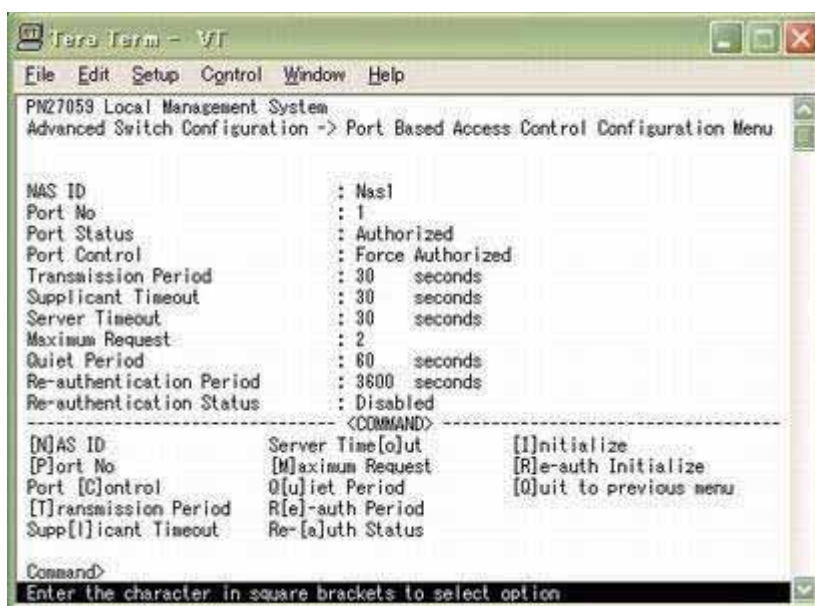
図4-7-9 IEEE802.1Xポートベース認証機能の設定
