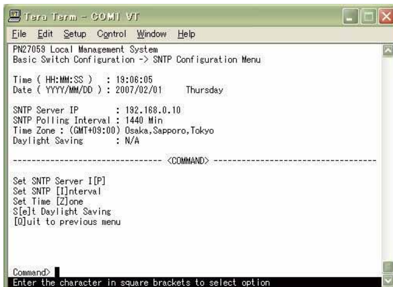
図4-6-20 時刻同期機能の設定設定後
