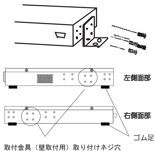
図2-4 壁面への取り付け
