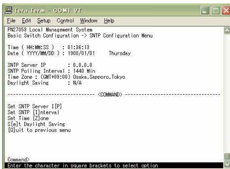
図4-6-19 時刻同期機能の設定
