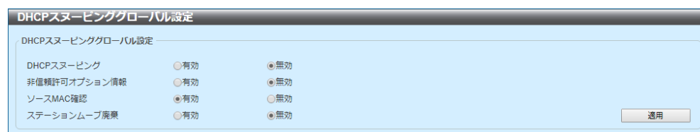
図 9-38 DHCP スヌーピンググローバル設定
