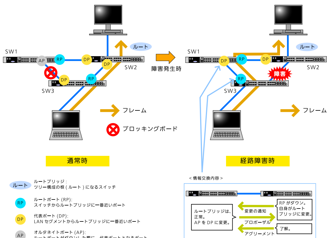
図 58-2 RSTP の概略
