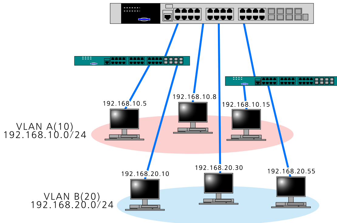
図 62-1 Subnet VLAN の概略
