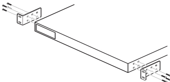
図 2-1 19 インチラックへの設置
