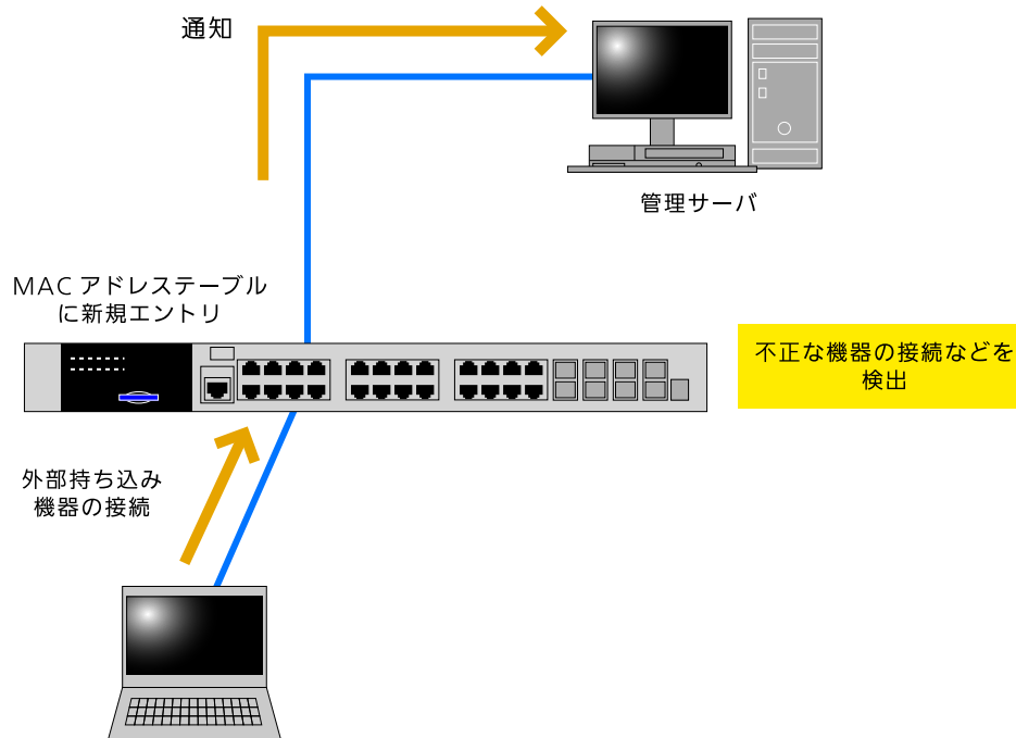
図 40-1 MAC Notification の概略
