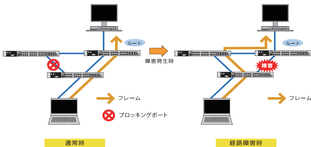
図 55-1 リングプロトコルの概要
