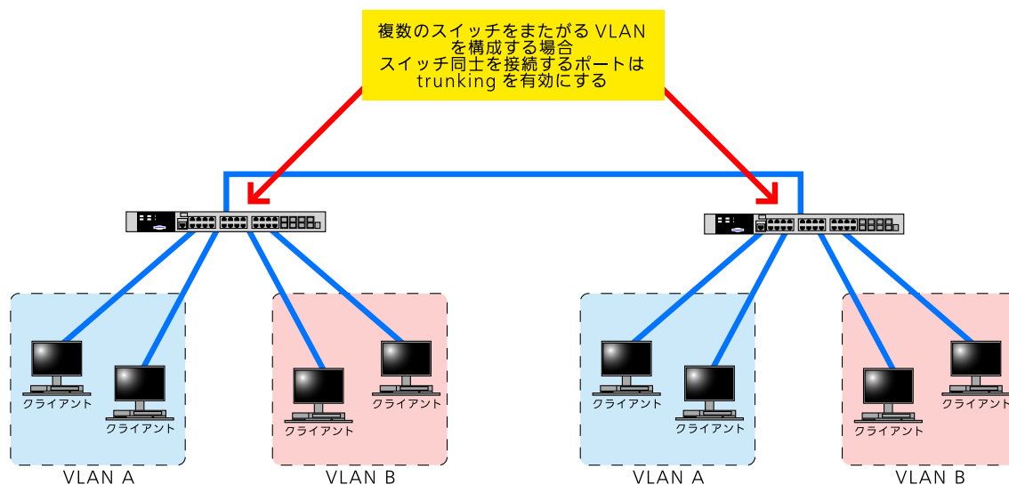
図 71-1 VLAN Trunking の概略
