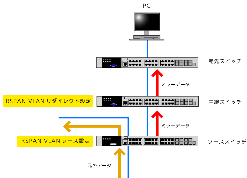
図 56-1 RSPAN の概略
