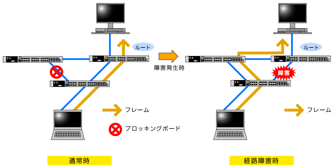
図 58-1 STP の概略
