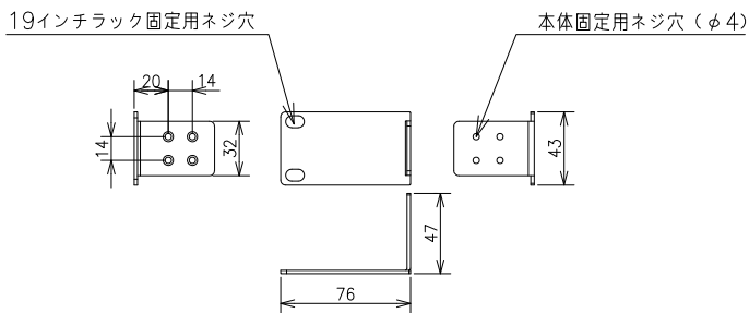
19インチラック固定用金具 (同梱)
