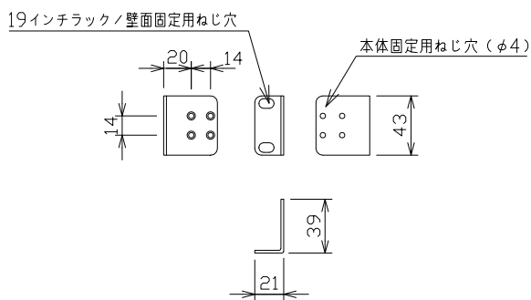
19インチラック固定用金具 (同梱)
