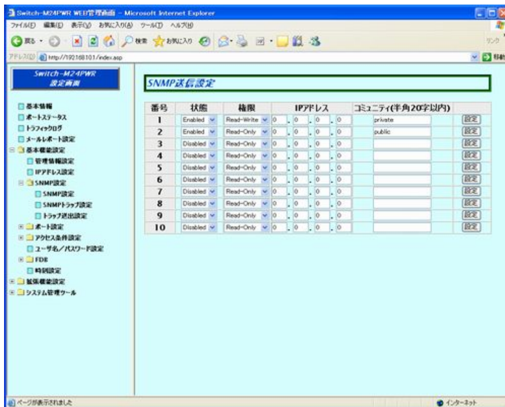
図 4-1-3 SNMP の設定
