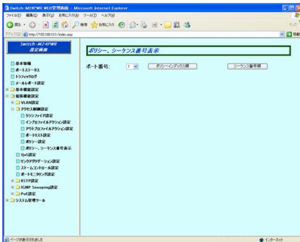
図 4-2-10 QoS 設定
