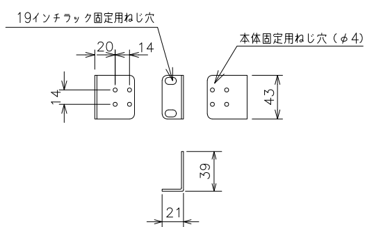
19インチラック固定用金具 (同梱)
