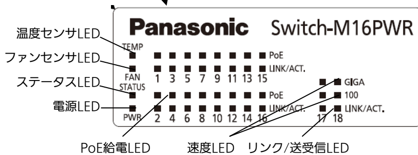
図1-2 前面LED拡大図
