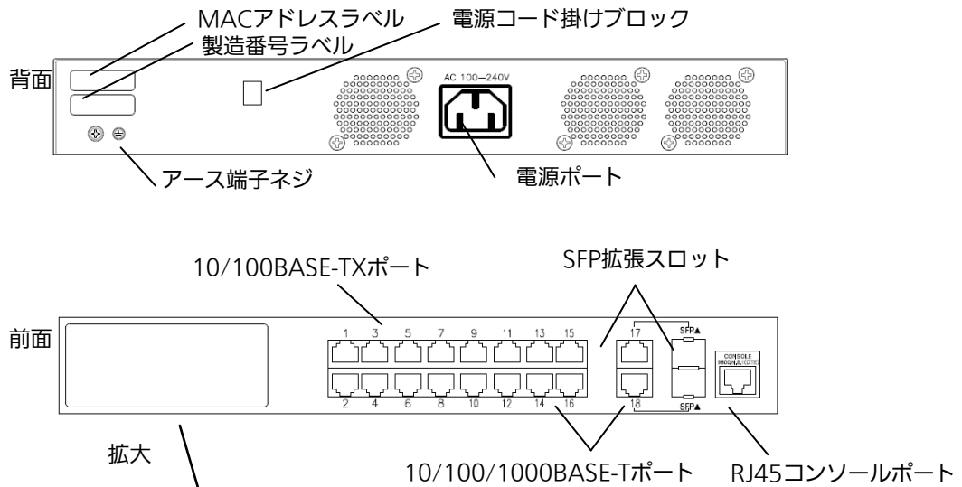
図1-1 Switch-M16PWR 外觀図
