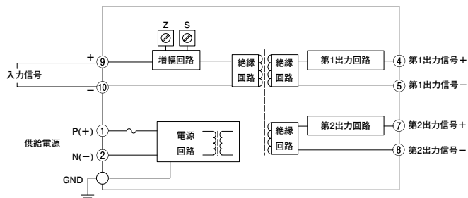
■ブロックダイアグラム 端子接続図
